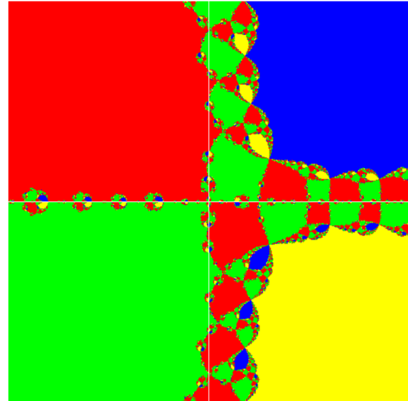
Το ίδιο fractal με βήμα 5\times μικρότερο.
